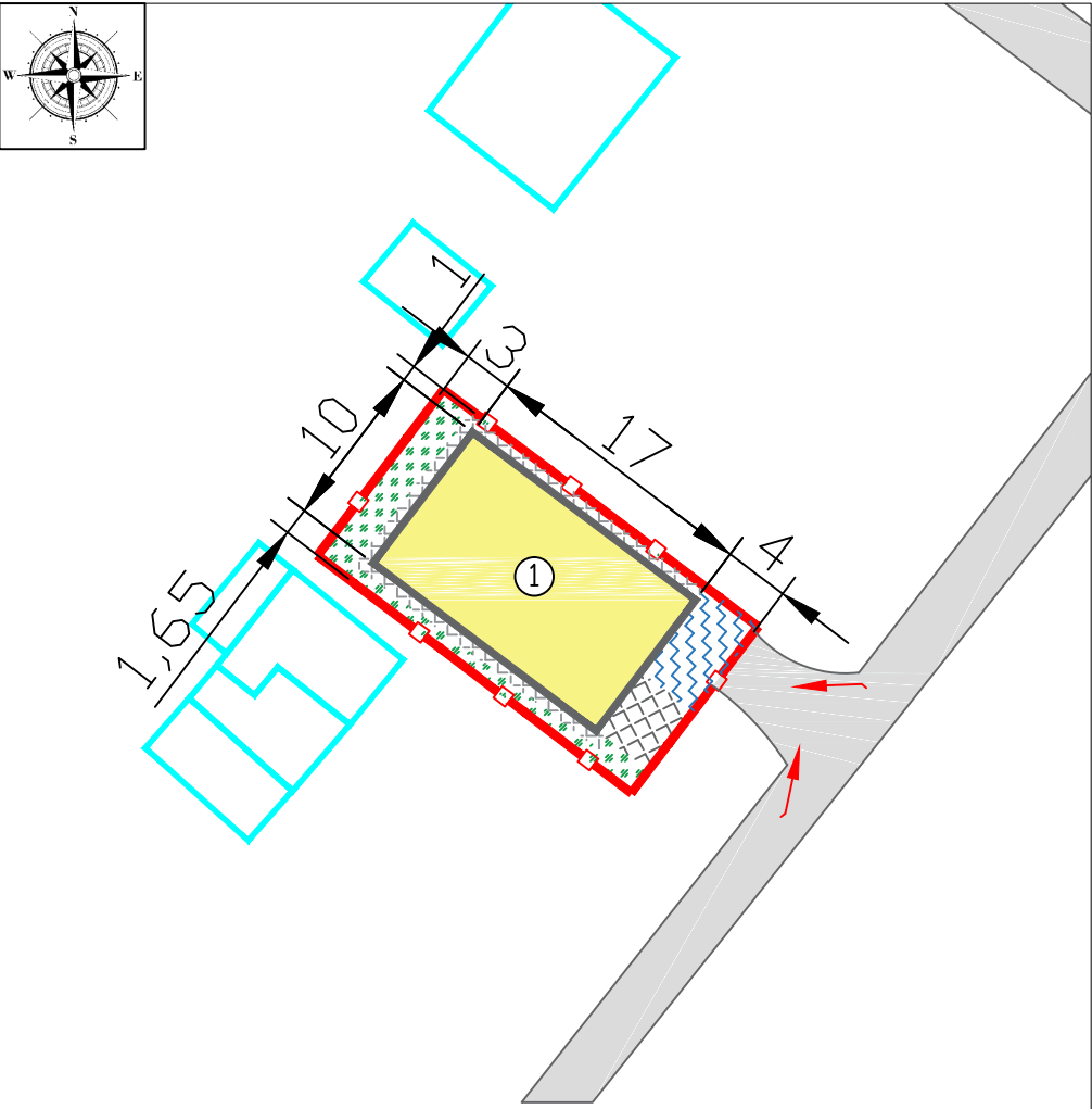
Генплан земельного участка М 1:500
