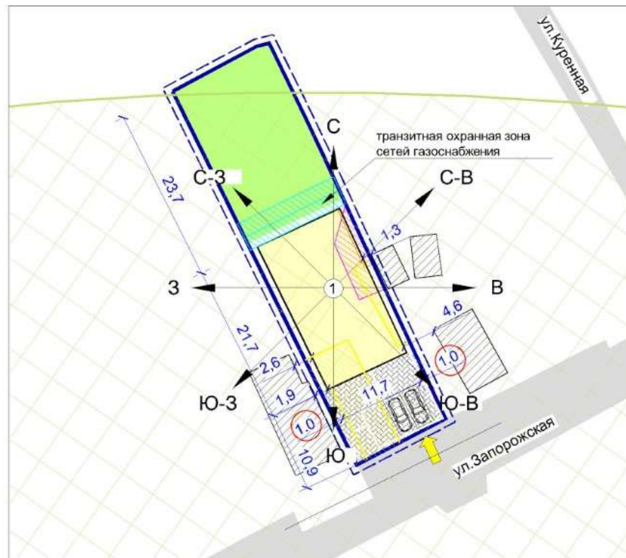
Технико-экономические показатели по земельному участку с кадастровым номером 23:43:0409007:110
