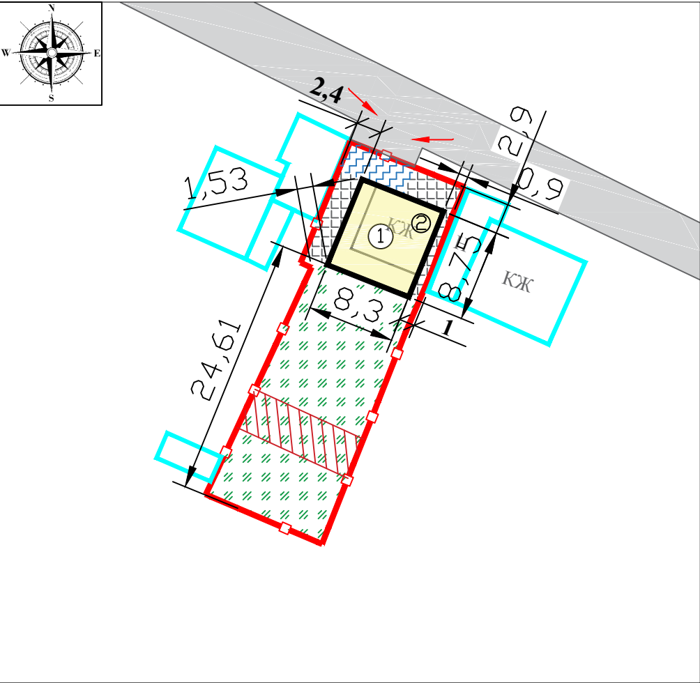
Генплан земельного участка М 1:500
